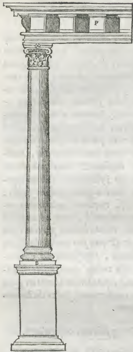
Composita integra columnatio, cum trabeatione.
